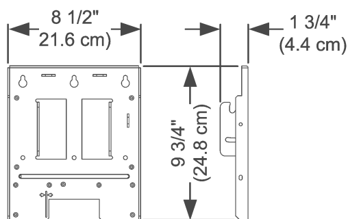
Montážna konzola - pohľad spredu
