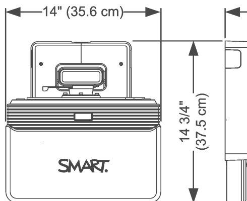
Interaktívny projektor - pohľad spredu
