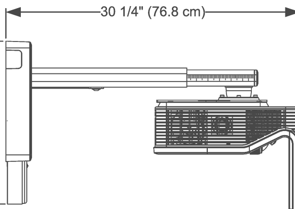
Interaktívny projektor - pohľad z boku
